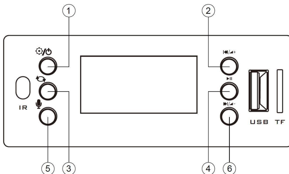
Рис. 3.10. Встроенный MP3 проигрыватель контроллера LPA-PRESTA-16.
