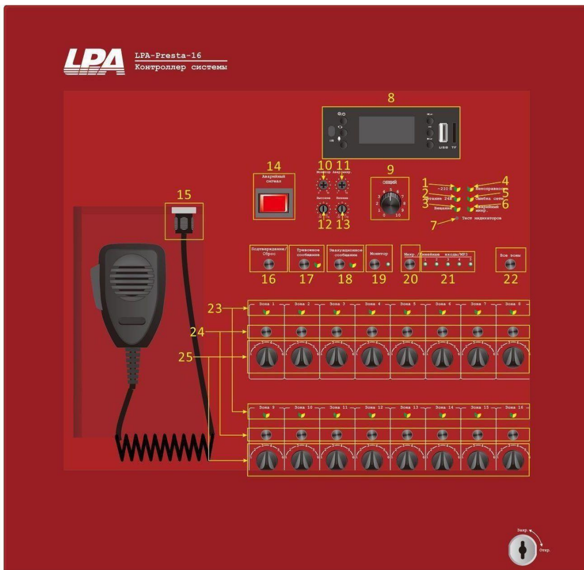
Рис. 2.1. Контроллер системы LPA-PRESTA-16 (передняя панель)
