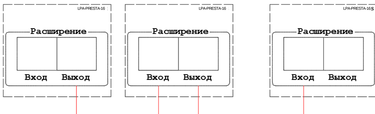
Рис. 3.6. Схема подключения блоков в системе LPA-PRESTA-16.
