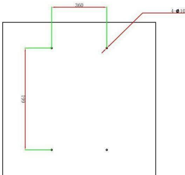
Рис. 3.7.1. Монтажные отверстия для LPA-Presta-16
