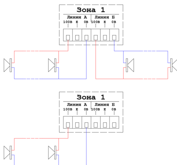
Рис. 3.2. Схема подключения трансляционных линий к LPA-PRESTA-16
