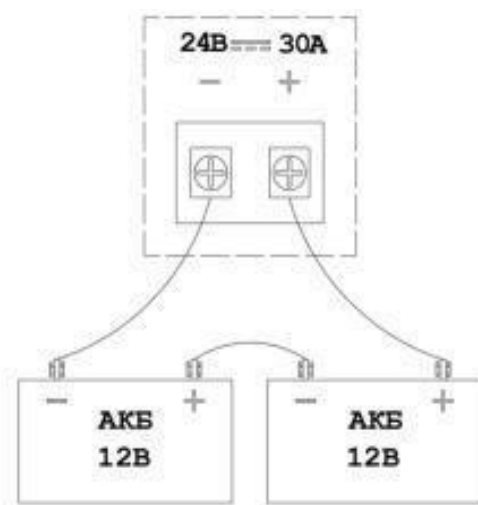
Рис. 3.1. Схема подключения АКБ к LPA-PRESTA-16
