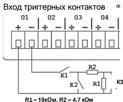
Рис. 3.3. Схема подключения внешних сигналов управления к LPA-PRESTA-16 с контролем целостности
