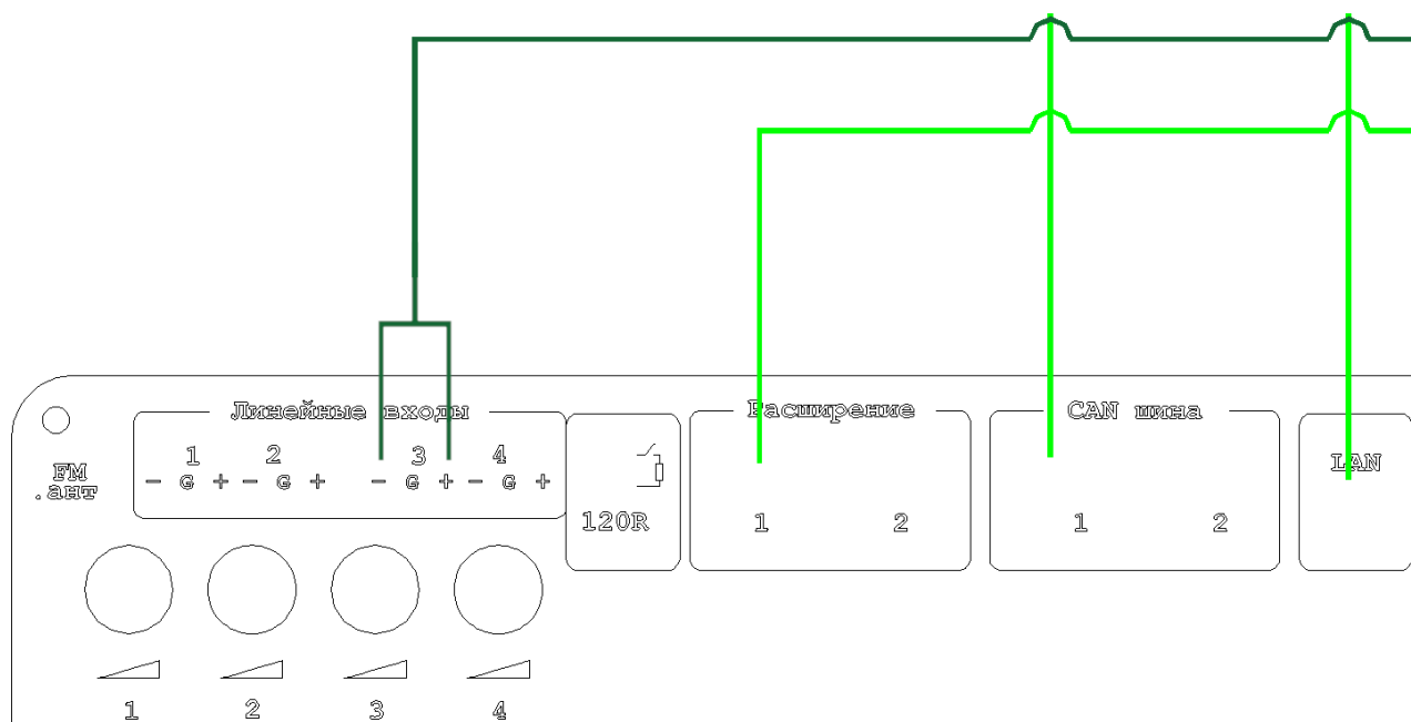
Рис. 3.8. Схема подключения сигналов ГО и ЧС к LPA-PRESTA-16.
