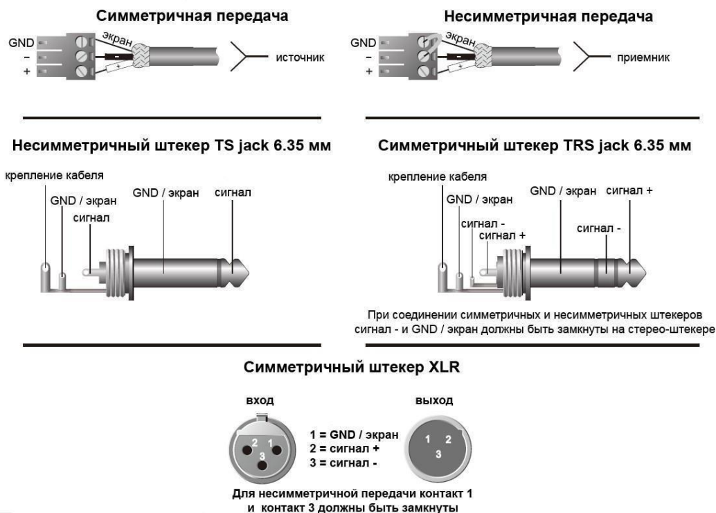
Рис. 3.11. Назначение контактов разъемов
