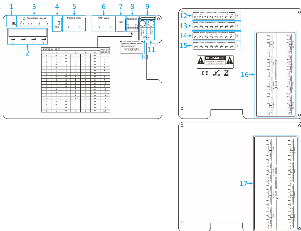
Рис. 2.2. Контроллер системы LPA-PRESTA-16 (внутренняя панель)
