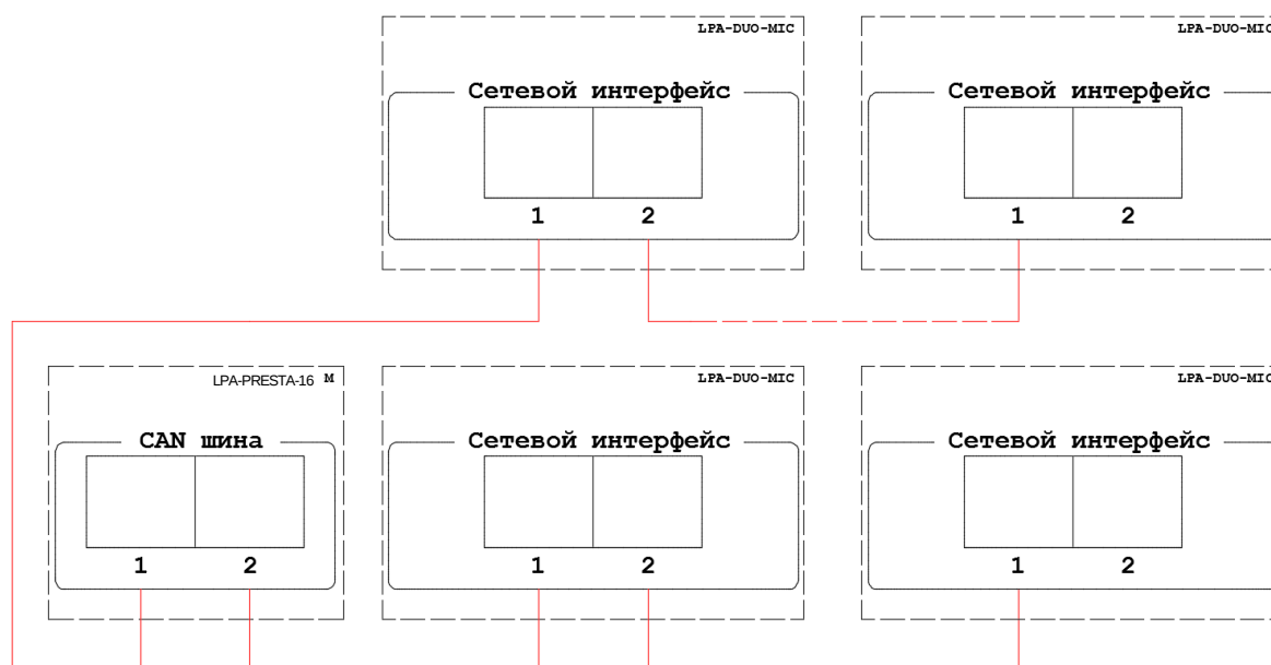
Рис. 3.7. Схема подключения удаленных микрофонных консолей к LPA-PRESTA-16.
