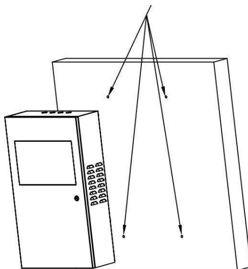
Рис. 3.7.2. Расположение LPA-Presta-16 на стене
